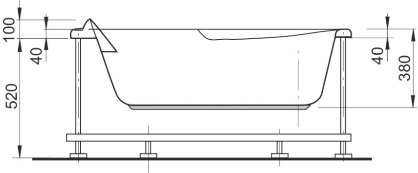
Presek "A-A"
